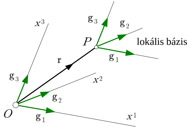
1.2. ábra. Ferdeszögű egyenesvonalú KR
