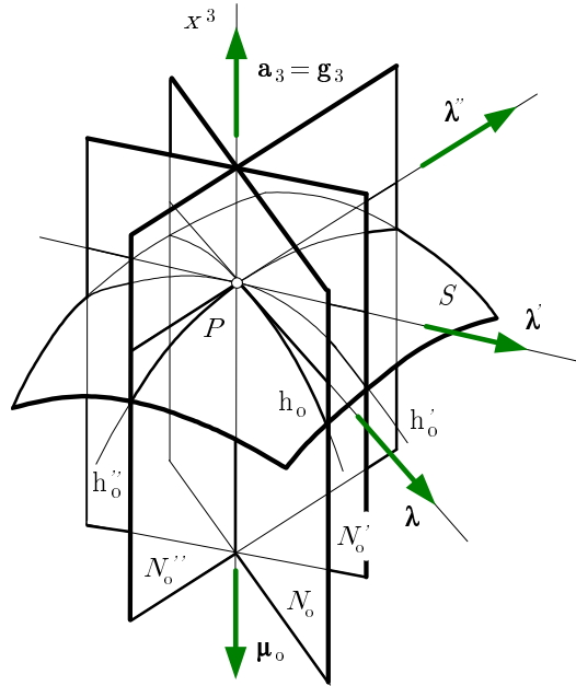
9.4. ábra. A felület normálisa körül forgatott síkok és a felület metszetei
